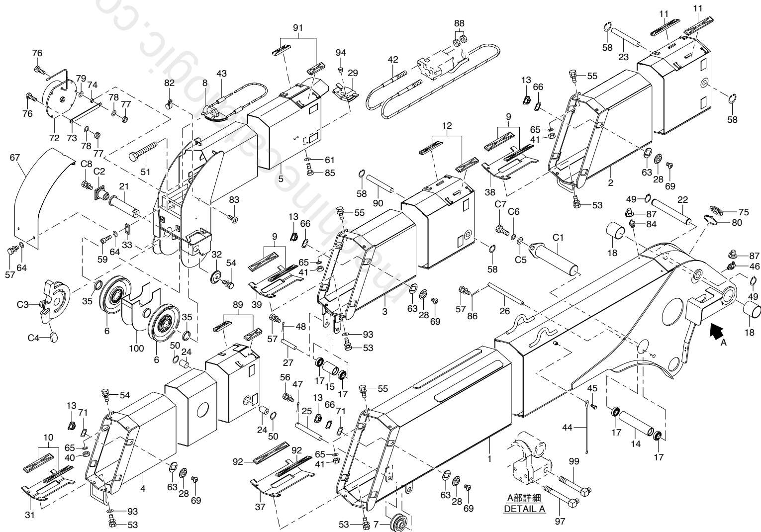
Fig. 1-6 5段ブーム組立 (URU375 R 仕様) 5-section BOOM ASS'Y (URU375 R type)
